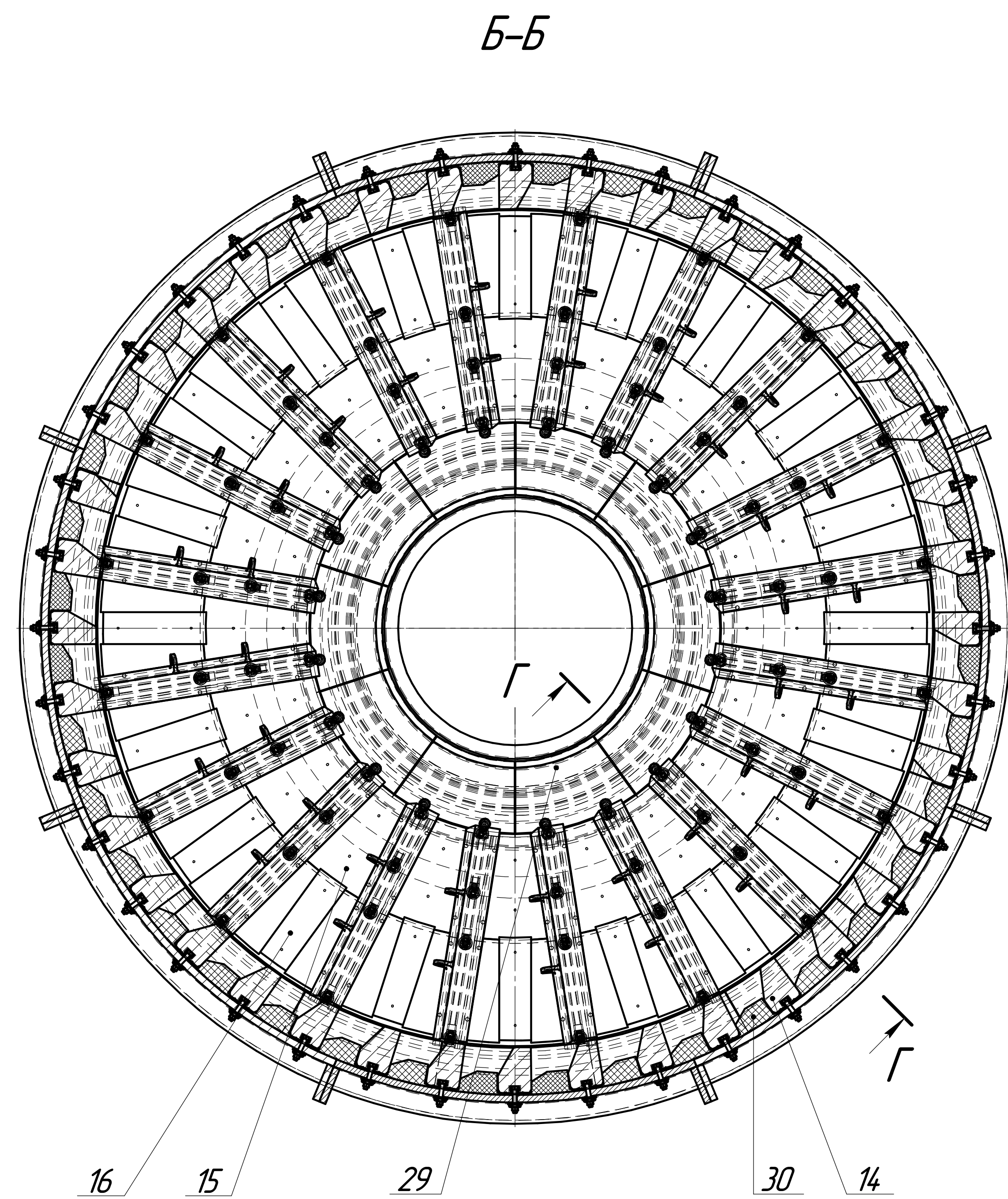
Г-Г(1:10)
