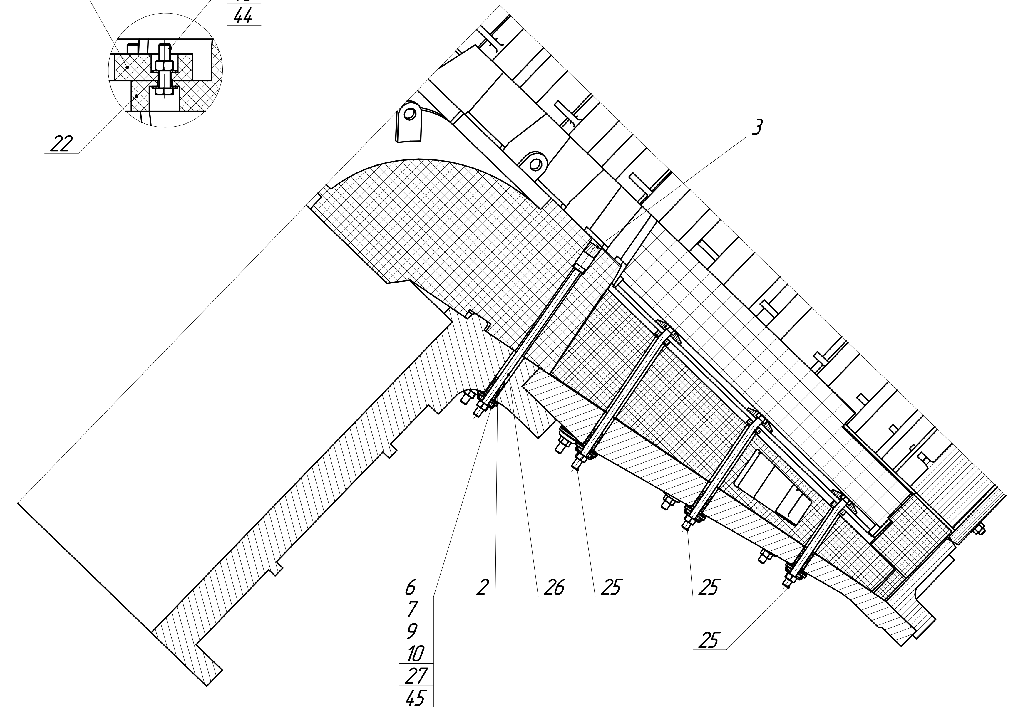
Е-Е(1:10)
